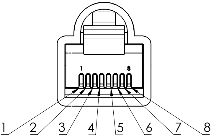
P2 RJ45
